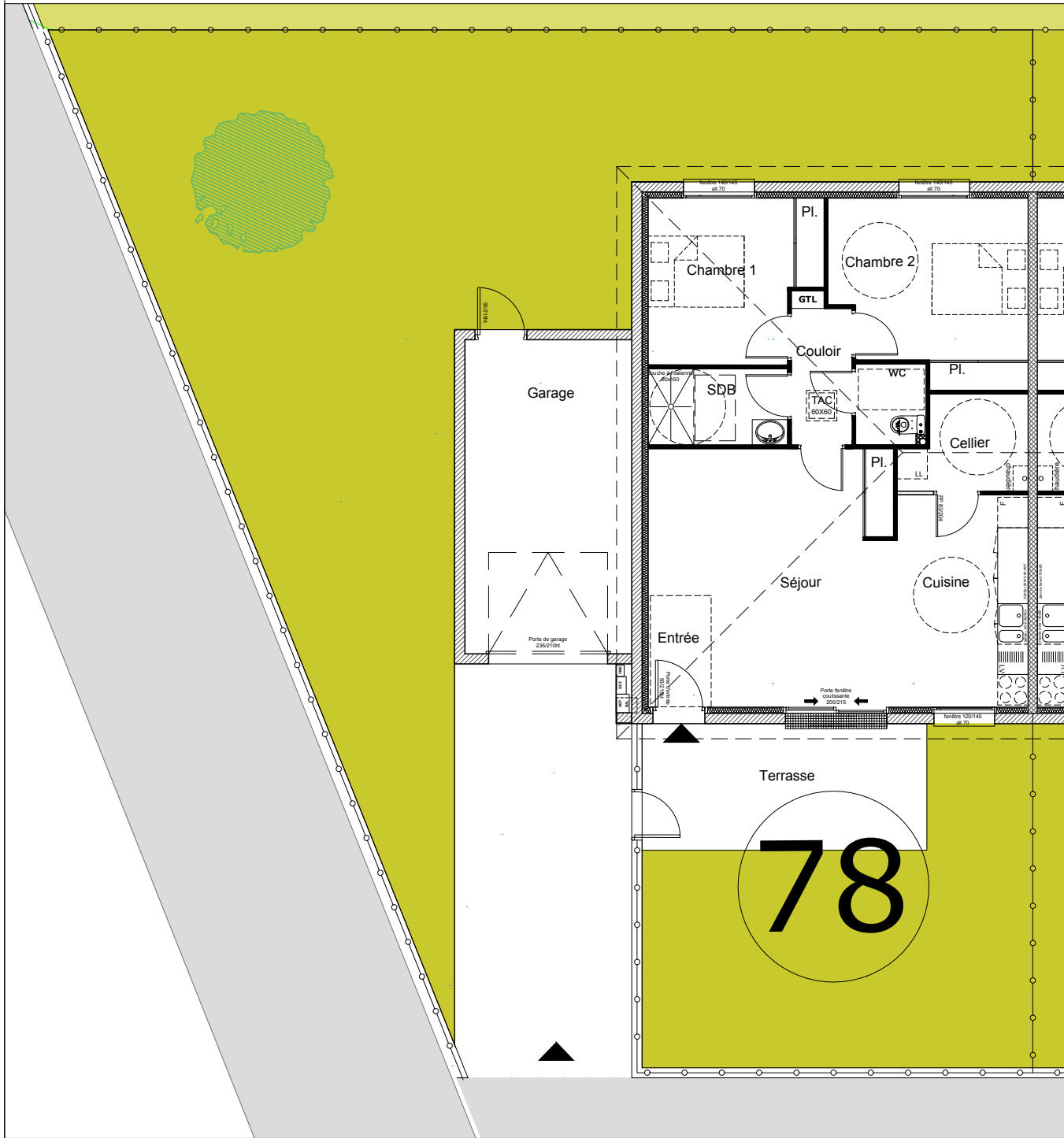
Rez-de-chaussée
